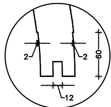
Detalle hembra
